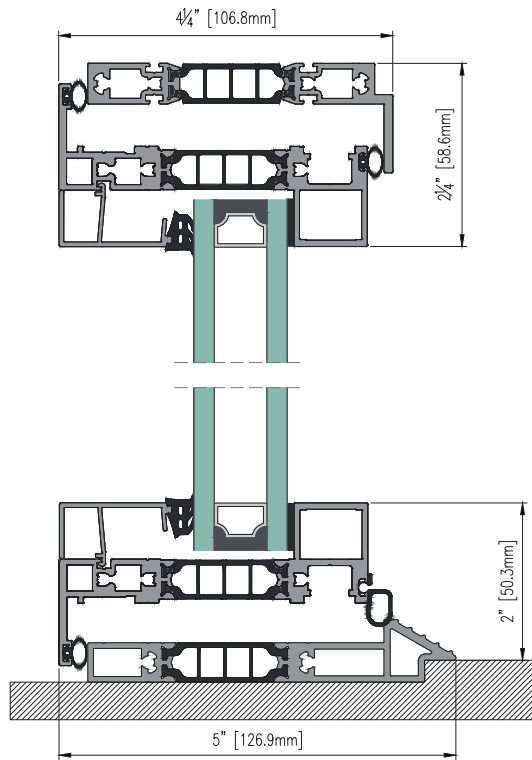
MOREVIEW INWARD OPENED DOOR
